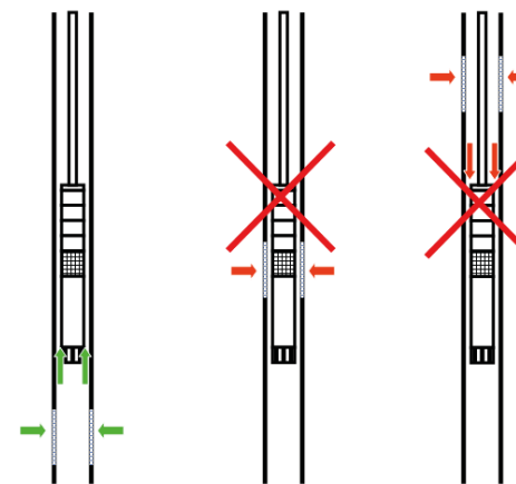
Instalando un equipo en un pozo (Figura 1.)
